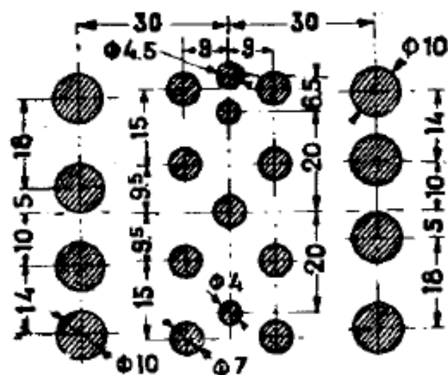
Foratura chassis
